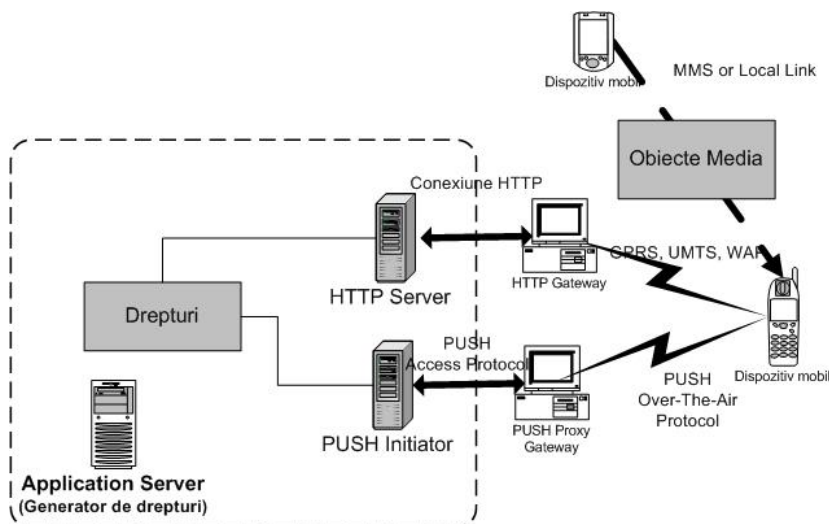
Fig. 4. Arhitectura super-distribuției.
